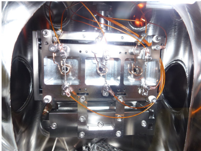
活性化chamber内部の写真
