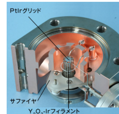
極高真空対応型残留ガス分析器
