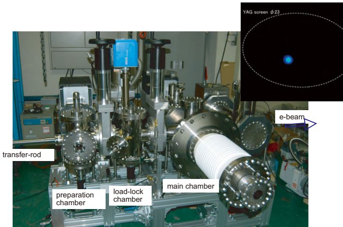
日本原子力研究開発機構 (JAEA) で開発された 250kV 電子銃。ビーム引き出し試験 (右上写真) に成功しました。
