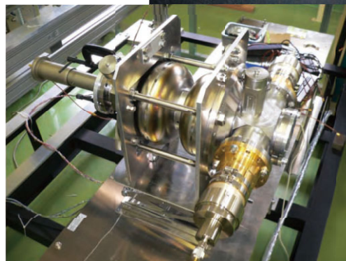
ERLの前段加速器で用いられる超伝導加速空洞。
