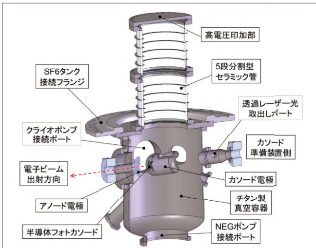
500kV 電子銃の全体図
