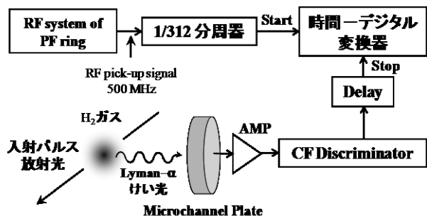
図 1: 実習装置の概略
