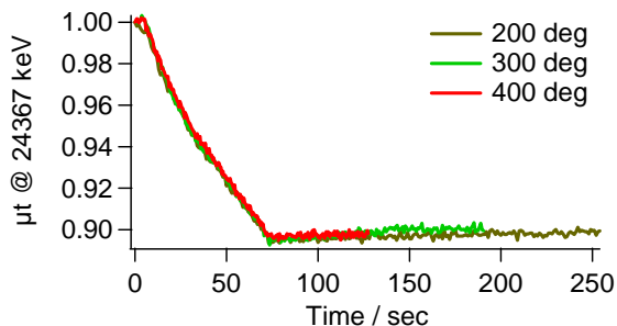
図 5 各温度における 24367 keV における吸光度変化
