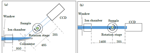
図1 (a)吸収コントラストCTの光学系 (b) Dual-Energy CTの光学系
