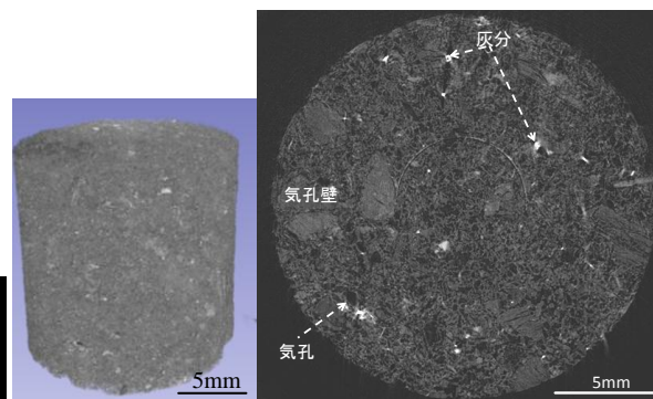
図 7 (左)コークスの 3 次元 CT 像
