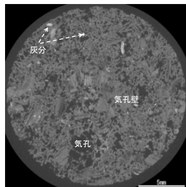
図 8 実験室線源 X 線 CT 装置によるコークスの断面図
