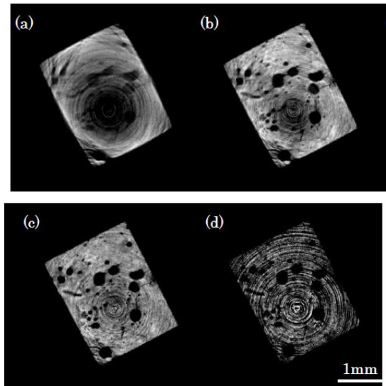
図5 焼結鈇(2mm)のXY断面図
