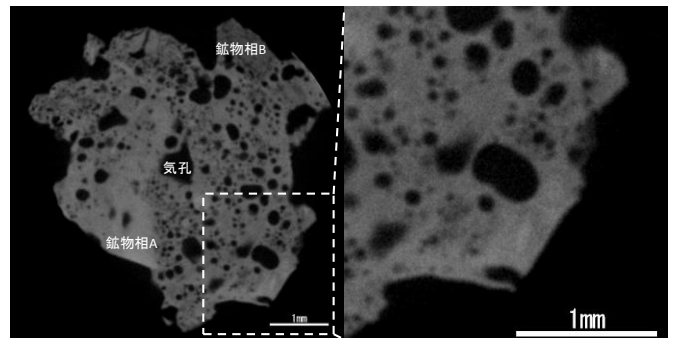
図4 実験室線源X線CT装置による焼結鈇の断面図
