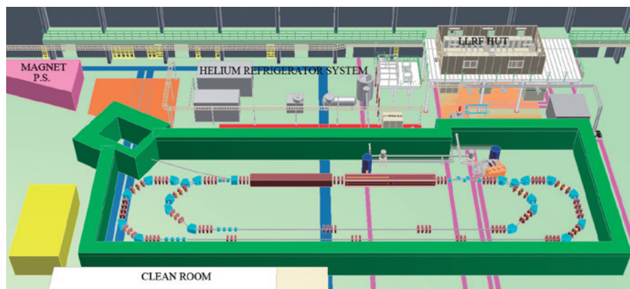
現在建設を進めているコンパクトERLの完成図
