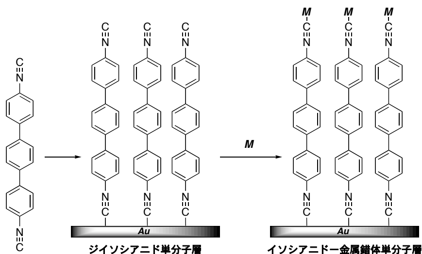
図1 金表面上のジイソシアニド-金属錯体単分子層の形成.
