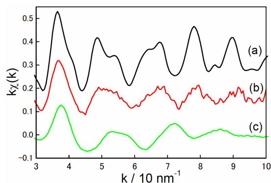
図 1 (a) Au foil、(b) \text{TiO}_2(110) 上に固定化した \text{Au}_{11} クラスタ、(c) \text{Au}_{11} クラスタ粉末の EXAFS スペクトル。
