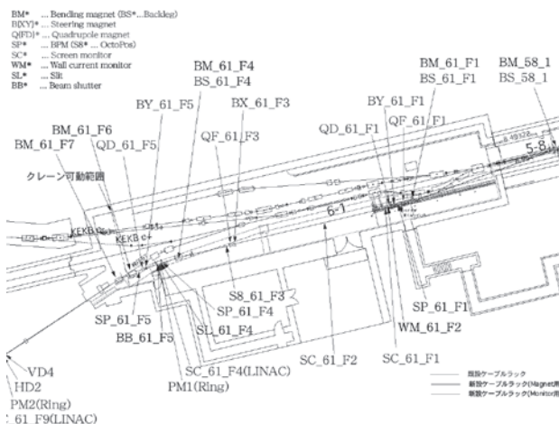
図1 入射器終端のビームスイッチヤード。入射器終端の#5-8加速モジュールが撤去され，その後にPFへの分岐電磁石BKが設置された。分岐後の入射ビームは新設のビームラインを輸送されスイッチヤード末端部でPF入射路に合流する。
