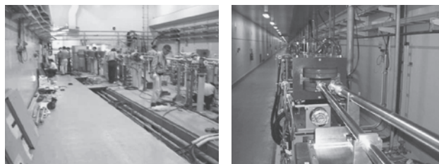
図2 入射器-PF入射路改善工事。左：夏期工事開始時。右：工事完成後のPFビーム分岐電磁石（BK 58_1 ）。
