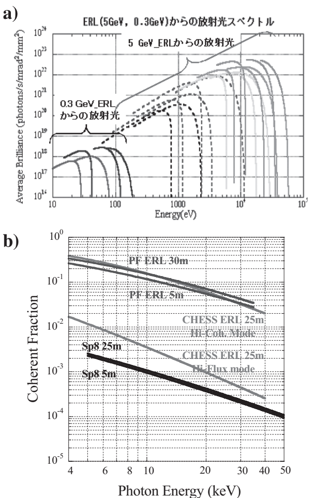
図2 ERL (5 GeV, 0.3 GeV)からの放射光の輝度およびコヒーレント・フラクション・スペクトル。a) 5 GeV ERLおよび0.3 GeV ERLに適切なアンジュレーターを用いることで数十 eVから数十 keVまでの放射光を得る。b) 軟X線からX線領域で期待されるコヒーレント・フラクション。10 keV領域で10～20%のコヒーレント・フラクションを達成。
