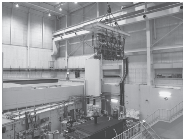
写真2 クレーンに宙吊りで運ばれるアンジュレータ
