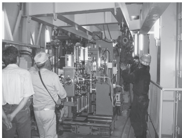
搬入作業中のNW14用真空封止アンジュレータ
