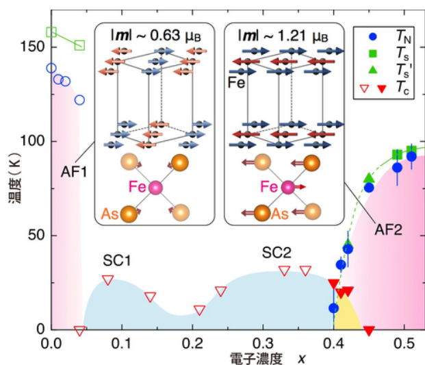
\text{LaFeAs}(\text{O}_{1-x}\text{H}_x) の電子状態相図 第二の超伝導領域 (SC2) に隣接して水素置換濃度 x が 0.4 を超えた領域で今回発見された第二の磁気秩序相 (AF2) が現れる。●がミュオン・スピン回転法・中性子回折により同定された磁気転移温度 (TN)、■、▲が放射光により同定された構造変化の温度 (TS, TS')。図の中央上段は中性子回折で同定された磁気構造。左上が x=0 の母物質中での磁気相 (AF1)、右上が今回見つけた新たな磁気相 (AF2)、矢印は \text{Fe}_2\text{As}_2 層で鉄イオンが持つ磁気モーメントの向きを示す。下段では構造変化に伴う鉄およびヒ素の原子位置の変化の向きと大きさを模式的に示した。(平石・他、DOI:10.1038/NPHYS2906)
