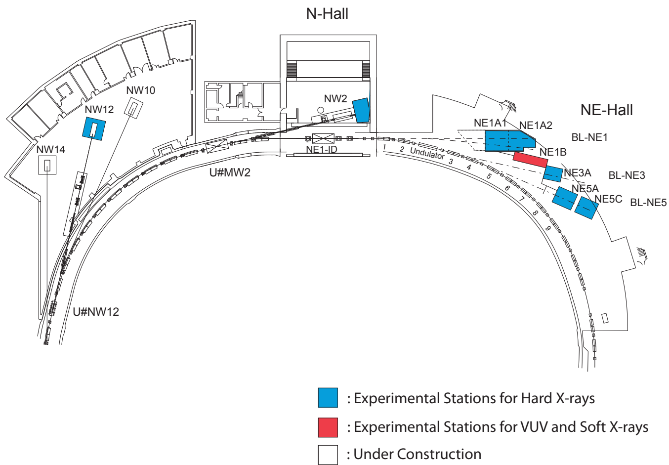
図2 (a) PFリングにおける2005年4月のBL状況
