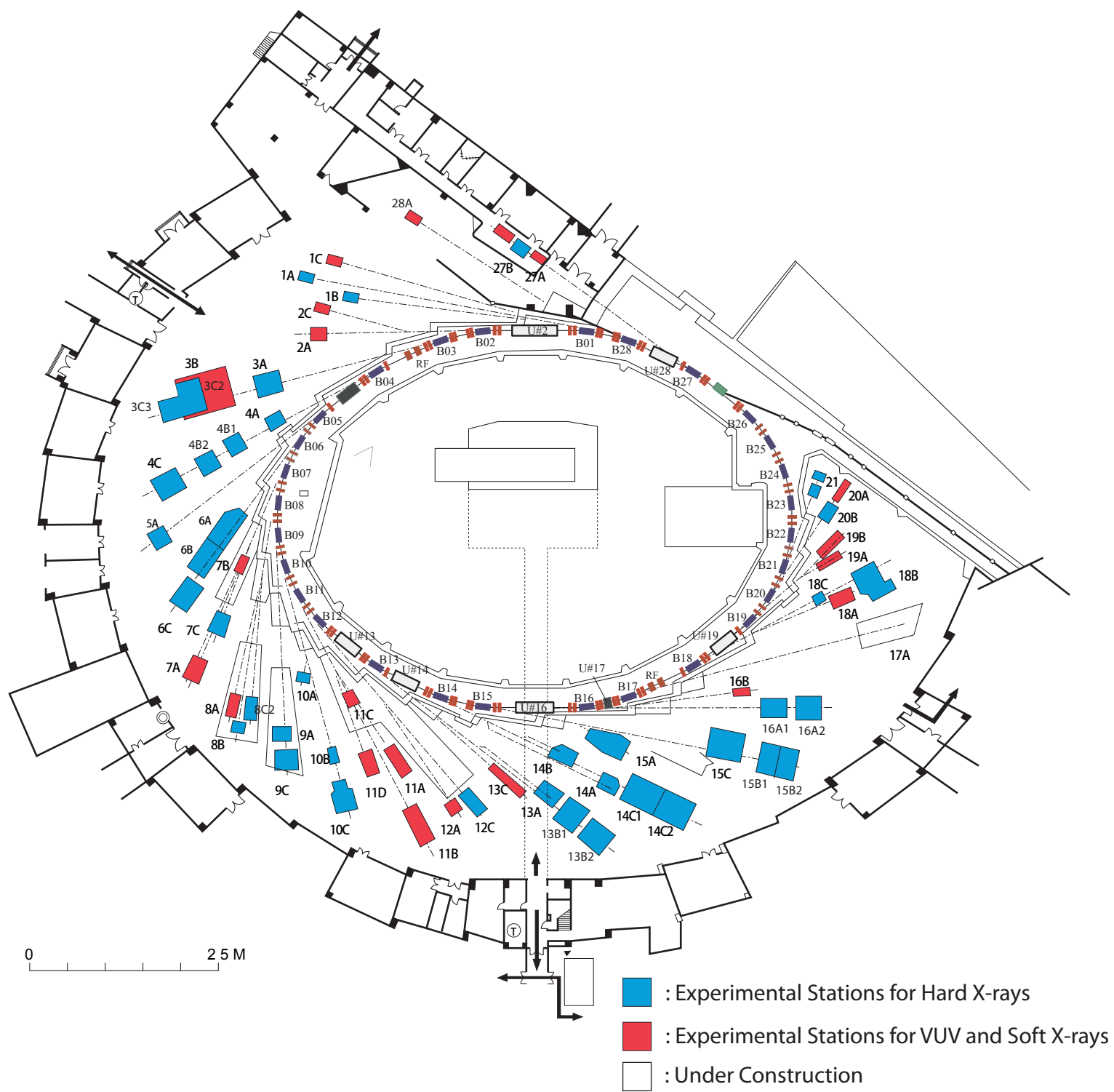
図1 (a) PFリングにおける2005年4月のBL状況
